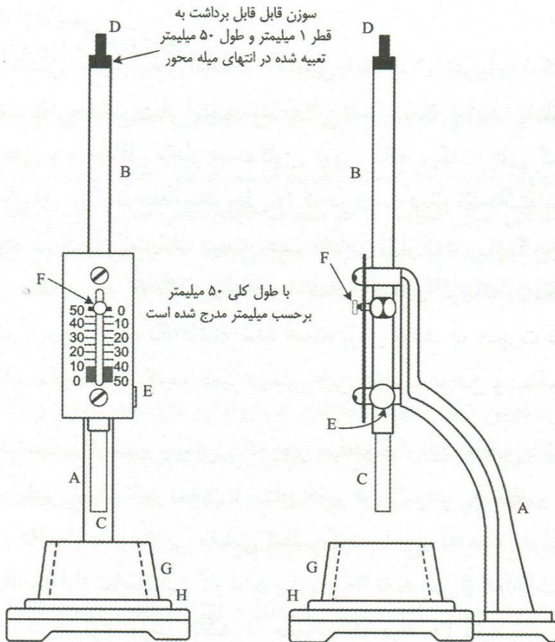
شکل ۱ دستگاه ویکات.
