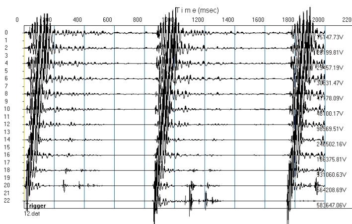
شکل ۶-۱۴- شمایی از ثبت داده لرزه‌ایی در طول ۲ ثانیه (برای دید مناسب دامنه داده‌ها به حداقل کاهش داده شده است)
