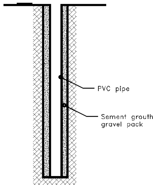
شکل ۶-۲- شمایی قرار گیری لوله PVC در گمانه و پر نمودن حاشیه خارجی آن
