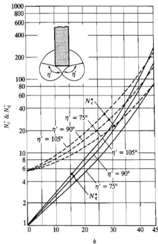
شکل ۷-۱۹ - نمودار تغییرات N_c^* و N_q^* با زاویه اصطکاک داخلی
