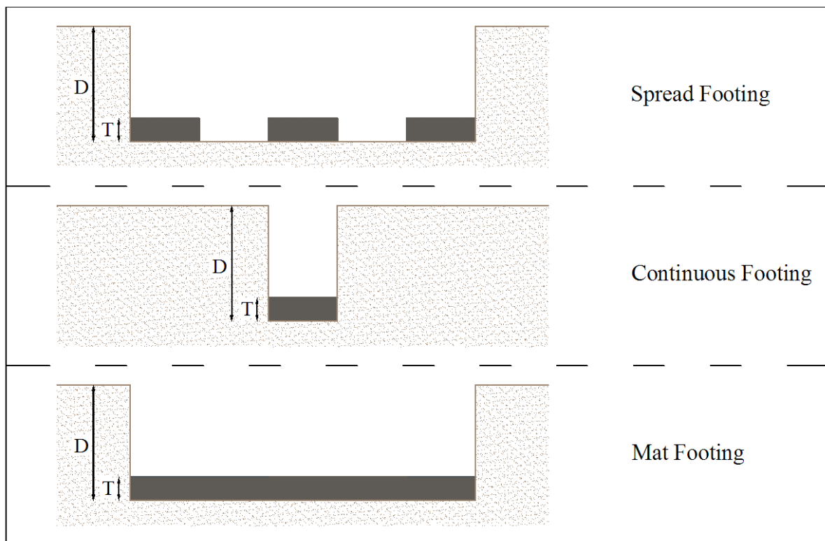
شکل ۷-۱ - نحوه آرایش شالوده های منفرد، یکپارچه و گسترده
