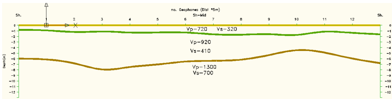
شکل ۶-۱۳- نمایی از مقطع نهایی برداشت ها روش شکسته مرزی
