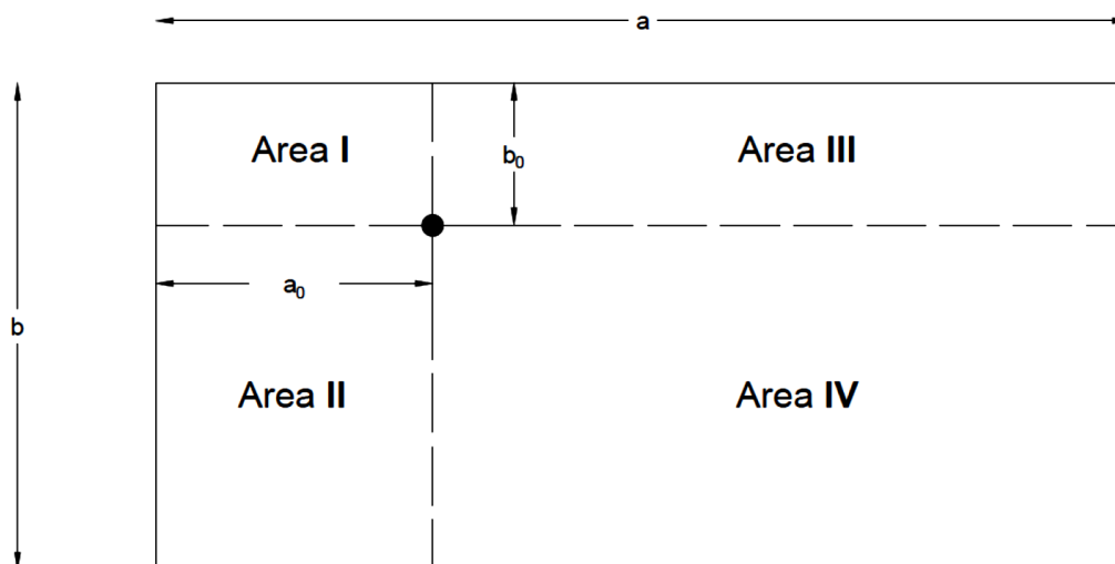
شکل ۹-۷- تقسیم بندی شالوده بر اساس نقطه مورد نظر
