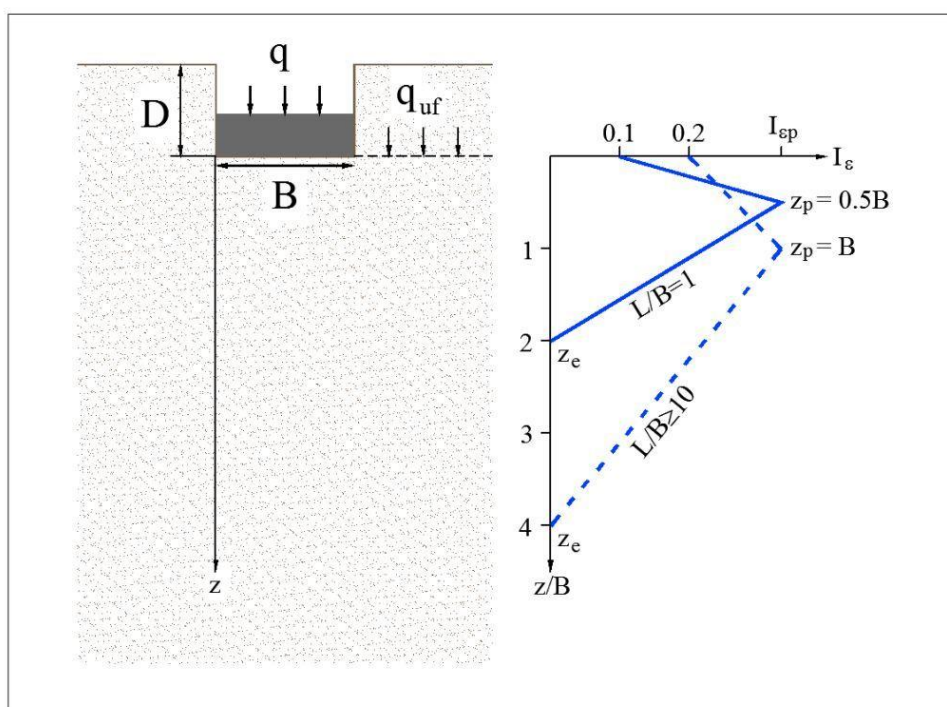
شکل ۷-۴ - تغییرات I_{\varepsilon} با عمق ( D ) و نسبت ابعاد پی ( L/B )
