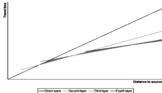
شکل ۳-۶- منحنی های زمان- مسافت یک مدل فرضی چهار لایه
