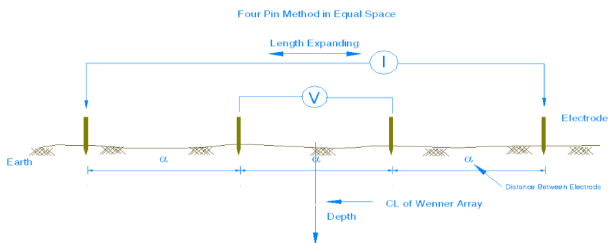
شکل ۶-۱- آرایش ژئوالکتریکی ونر، در این آرایه فاصله بین الکترودهای جریان پتانسیل یکسان می باشد
