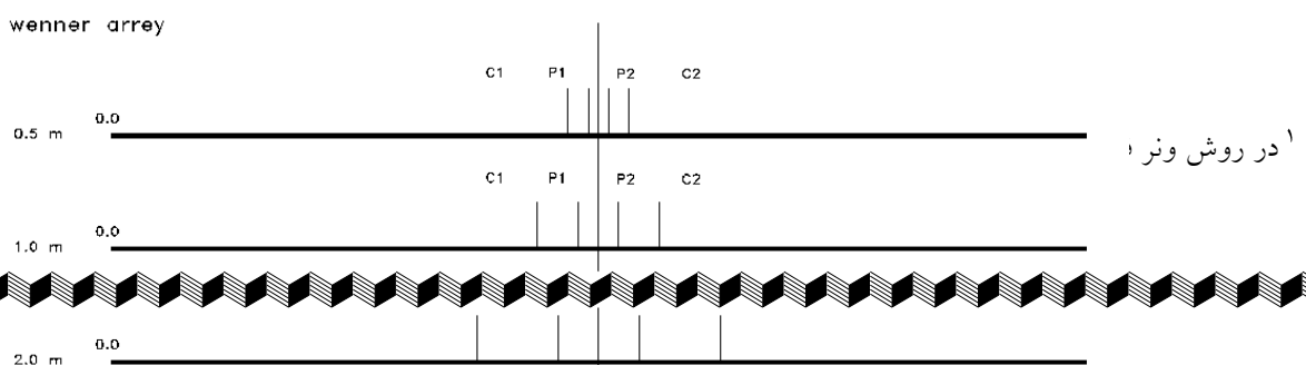
شکل ۶-۱- آرایش ژئوالکتریکی ونر، در این آرایه فاصله بین الکترودهای جریان پتانسیل یکسان می باشد
