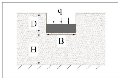
شکل ۳-۵ - پارامترهای مورد استفاده در روش جانبو
