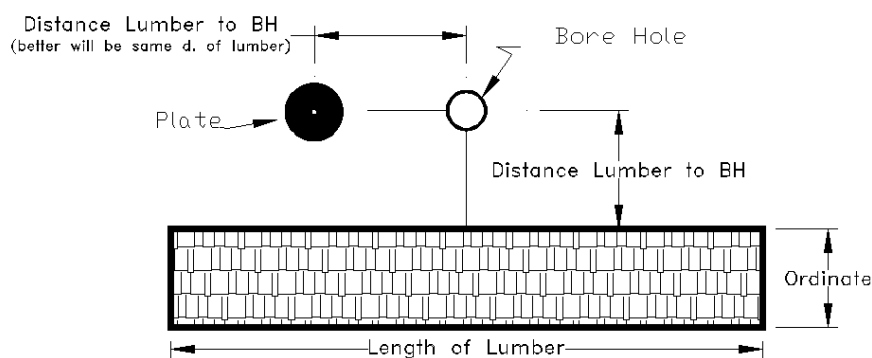
شکل ۶-۳- شمایی پیگیربندی برای برداشت لرزه نگاری
